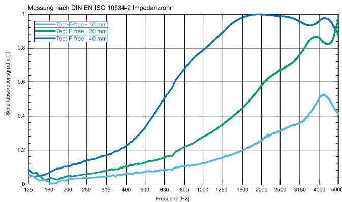
Schallabsorption nach DIN EN ISO 10534-2
